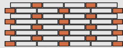
ЦЕПНАЯ КЛАДКА
