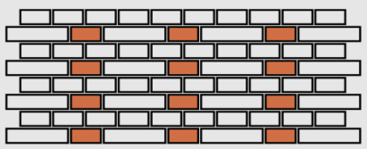
ГОЛЛАНДСКАЯ КЛАДКА
