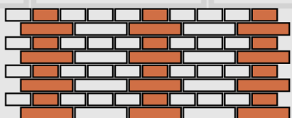
БРАНДЕРБУРГСКАЯ КЛАДКА
