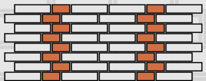
СИЛЕЗСКАЯ КЛАДКА
