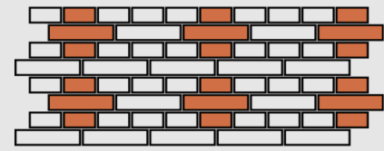
КРЕСТОВАЯ КЛАДКА
