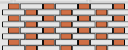
ФЛАМАНСКАЯ КЛАДКА
